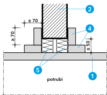
Detail B - průstup potrubí stěnou
