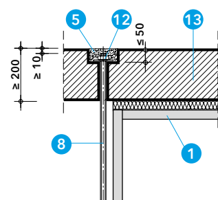
Detail C - připojení ke stěně
