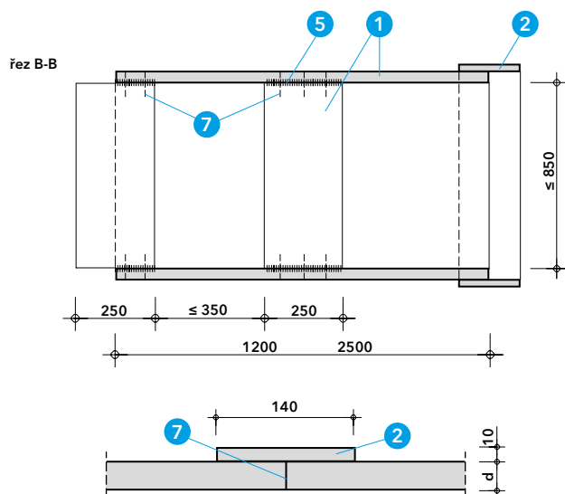
Objímka u velkých průřezů
