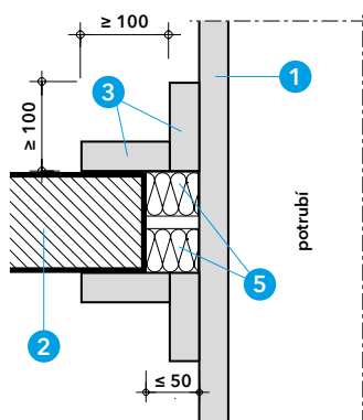
Detail C - průstup potrubí stropem
