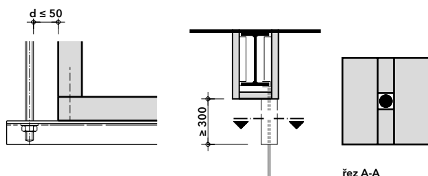
Detail C - závěsy
