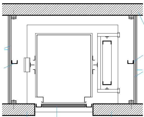
Detail A - výtahová šachta s ocelovými hrázďenými stěnami PROMATECT®-H, katalogový list 450.81
