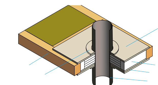
Detail C – prostup kouřovodu hořlavým stropem
