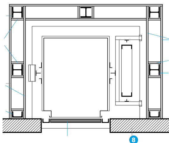
Detail A - výtahová šachta s ocelovými hrázďenými stěnami PROMATECT®-H, katalogový list 450.81
