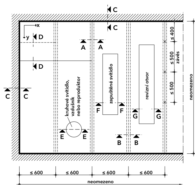
Detail A - stropní podhled
