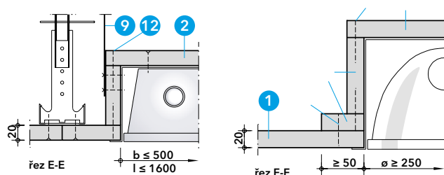
Detail F - vestavěné svítidlo
