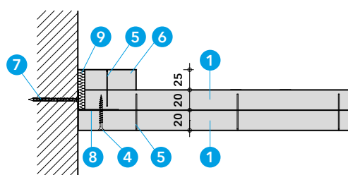
Detail A - s nosným T profilem
