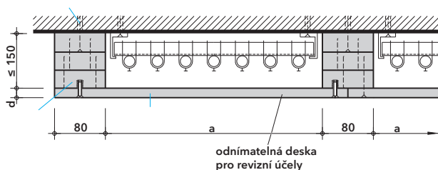
Detail F - nástěnný nebo stropní kanál
