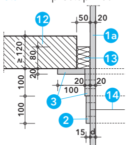
Detail E.2 - průstup stropem
