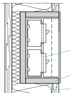
Detail D - malý rozvaděč v dřevěné stěně
