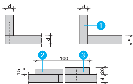
Detail D - rohový spoj a spojení pomocí objímky
