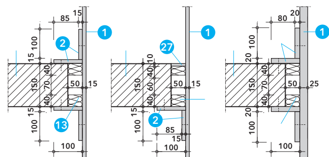
Detaily F.3 a F.4 - průstupy stropem
