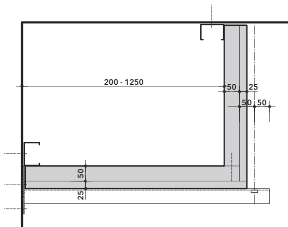
14 Detail B - dvoustranný přisazený kanál - řez
