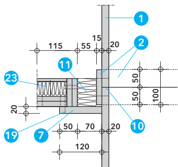
Detail E.3b - lehký strop
