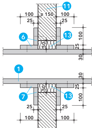
Detail F.1 - průstup stěnou
