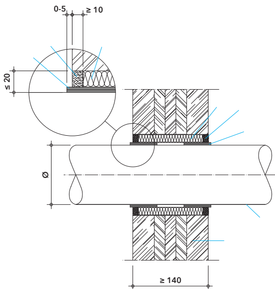
Detail C - vstup plastového potrubí s pásem PROMASTOP®-W v masivním stropě
