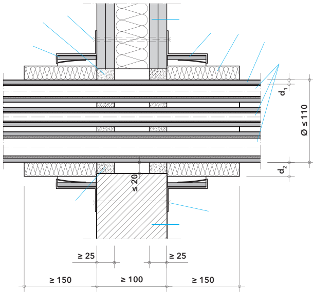
Detail I - průstup izolovaných vícevrstevných plastových potrubí s AL jádrem a přidanou nehořlavou izolací stěnou
