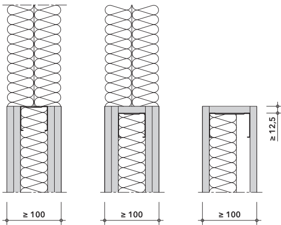
Detail D - provedení ostění otvoru v lehké příčce
