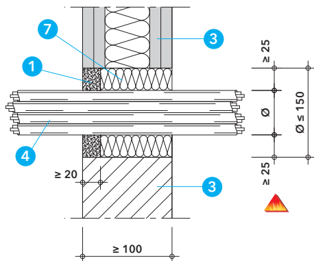
Detail C - vstup kabelů a kabelových svazků podle tabulky 2 v lehké přičce nebo masivní stěně
