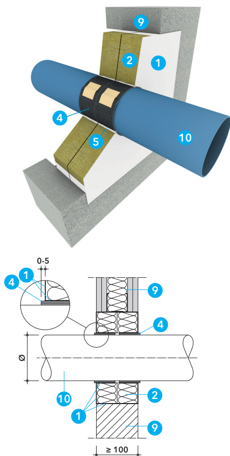
Detail V - vstup plastového potrubí ve stěněch 2)
