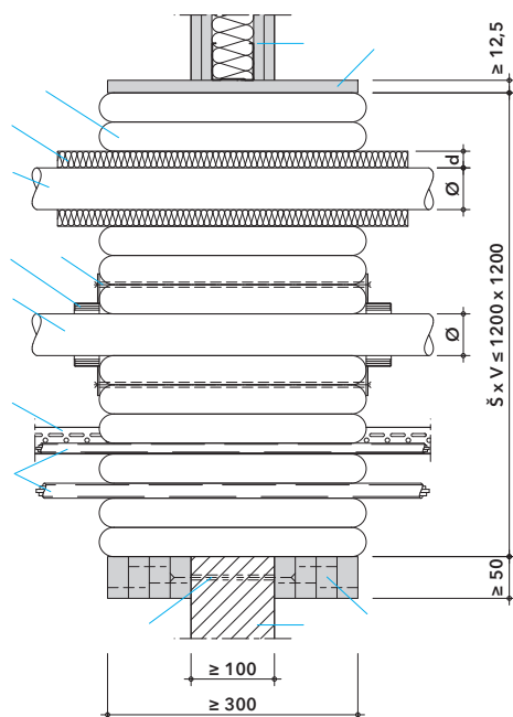
Detail A - kombinovaná přepážka PROMASTOP®-S/-L v lehké příčce nebo masivní stěně
