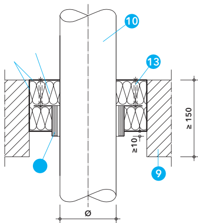
Detail P – vstup plastového potrubí ve střepech 2) – zapuštěná varianta
