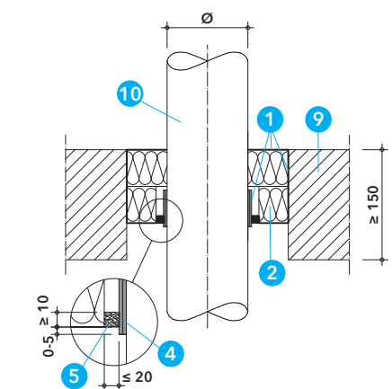
Detail W - vstup plastového potrubí ve stropěch 2)
