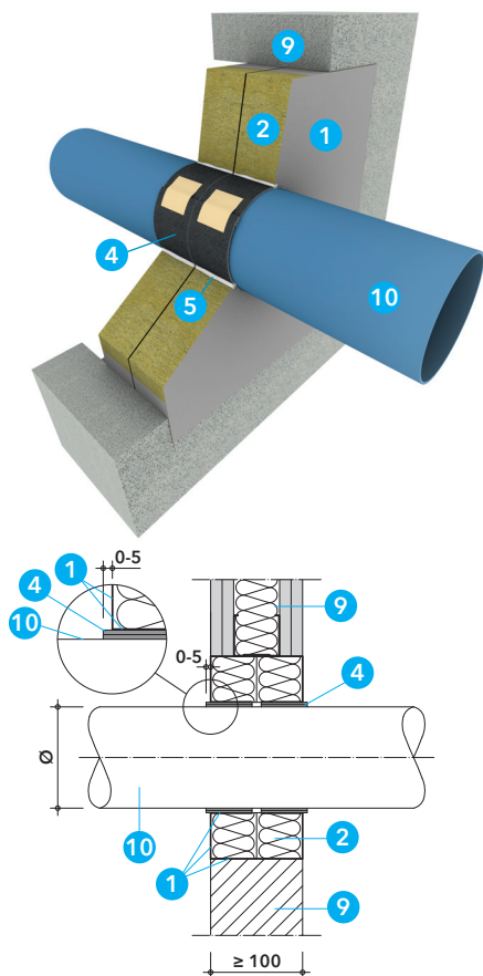
Detail S - průstup plastového potrubí bez izolace ve stěnách 2)
