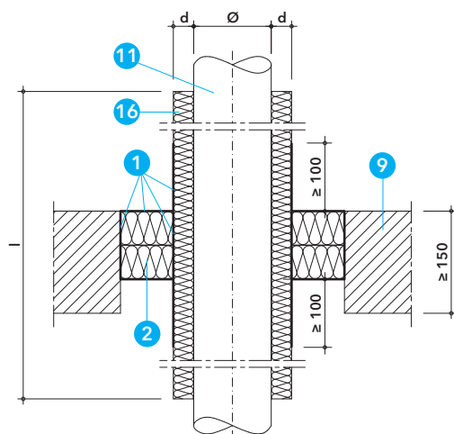
Detail J - vstup kovového potrubí přepážkou PROMASTOP®-CC ve stropech 1)
