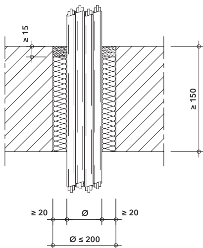
Detail A - vstup kabelů a kabelových svazků podle tabulky 1 v lehké příčce nebo masivní stěně
