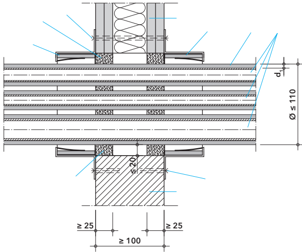
Detail H - průstup izolovaných vícevrstevných plastových potrubí s AL jádrem stěnou
