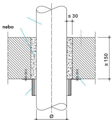
Detail G - vstup plastového potrubí v masivním stropě s manžetou
