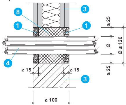
Detail E - vstup kabelového svazku podle tabulky 3 v lehké přičce nebo masivní stěně
