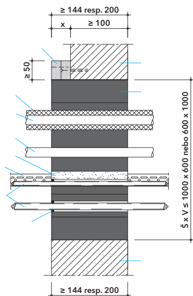
Detail B - kombinovaná přepážka PROMASTOP®-FB pro kabely a trubky v masivní stěně
