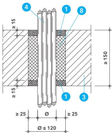
Detail F - vstup kabelového svazku podle tabulky 3 v masivním stropě
