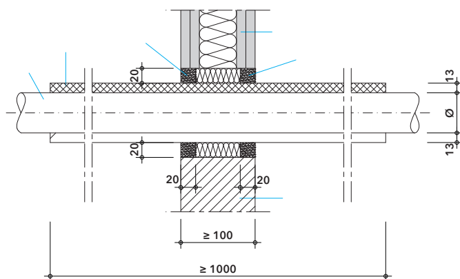
Detail O - prostup kovového potrubí podle tabulky 9 v lehké přičce nebo masivní stěně
