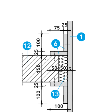
Detail E.3 - průstup stropem
