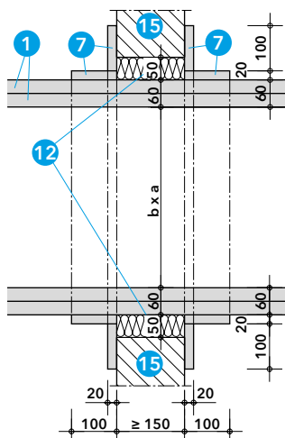
Detail D - průstupy stavební konstrukcí - řez
