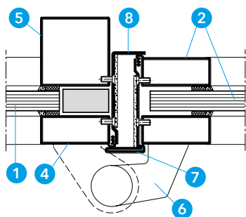
Detail C - řez A-A 270
