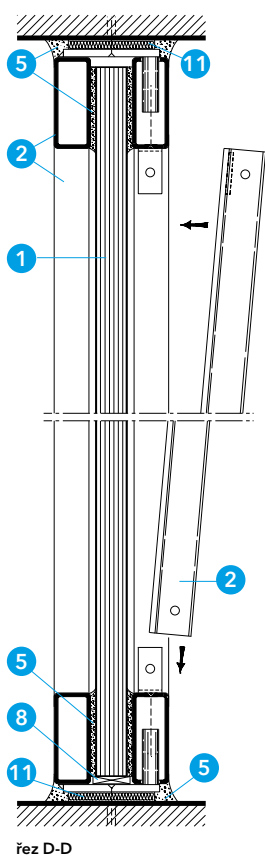
Detail B - svislý řez
