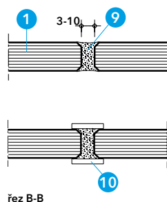
Detail D - spáry mezi skly
