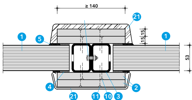
řez C-C
