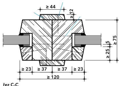
Detail D - spojení dvou ráků
