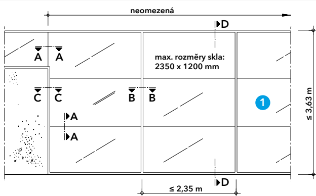
10 Detail A - rozměry
