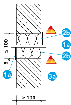
Detail I - vodorovná spára ve svislé konstrukci
