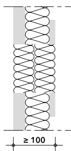
Detail M - spára v lehké šachtové příčce 236
