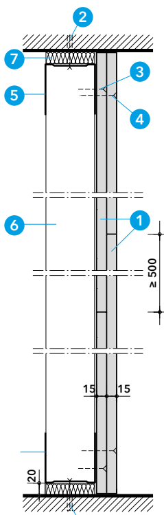
řez C-C
