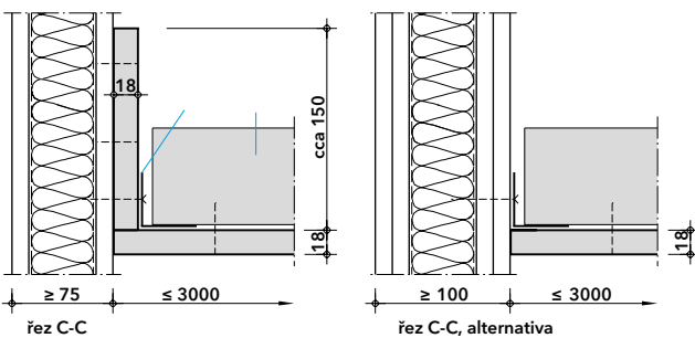
Detail F - připojení k lehkým příčkám \geq E1 30
