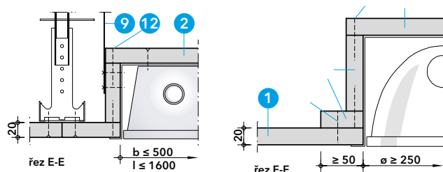
Detail F - vestavěné světlo
