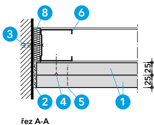
řez A-A
