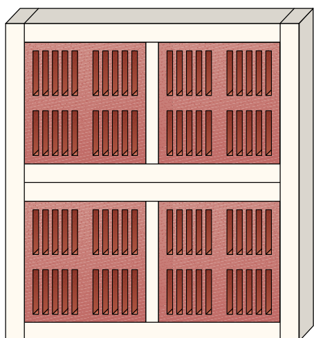
Detail B - sestava větracích tvarovek 2 x 2, 226 x 246 mm
