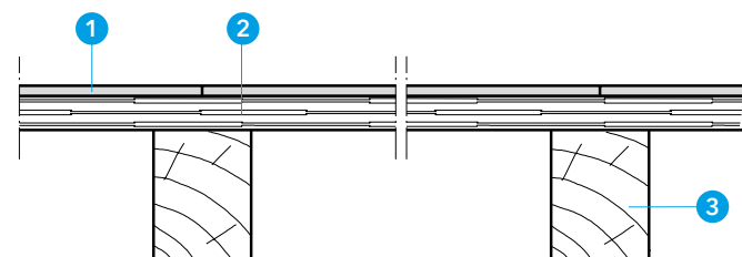
Dřevěný záklop
