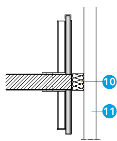
Detail D - požární utěsnění
