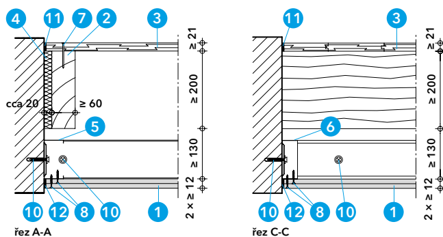
Detail B - napojení na stěnu
