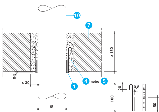
Detail C - průstřeh plastového potrubí s pásem PROMASTOP®-W v masivním stropě
