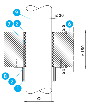
Detail F - průstup plastového potrubí v masivním stropě s manžetou PROMASTOP®-FC a tmelem PROMASEAL®-A
