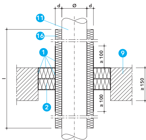
Detail J – prostup kovového potrubí přepážkou PROMASTOP®-CC ve stropě 1)
