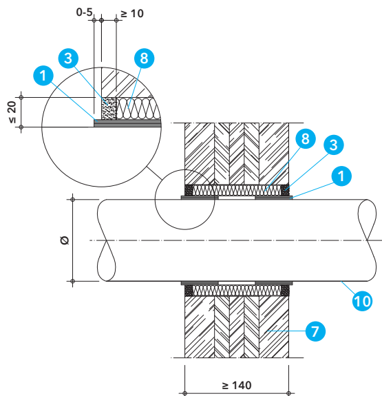
Detail E - průstřeh plastového potrubí s pásem PROMASTOP®-W v dřevěné stěně
