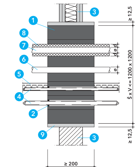
Detail A - kombinovaná přepážka PROMASTOP®-B pro kabely a trubky v lehké příčce nebo masivní stěně
