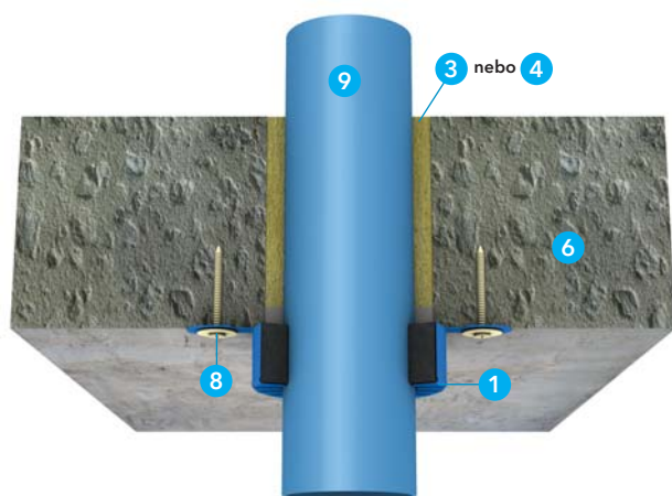
Detail A - prostup plastového potrubí s přisazenou manžetou PROMASTOP®-FC v masivním stropě
