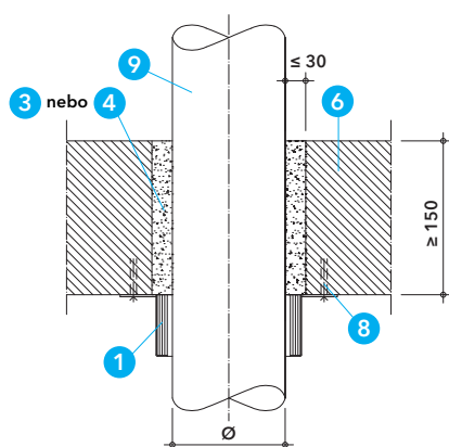
Detail G - průstup plastového potrubí v masivním stropě s manžetou PROMASTOP®-FC a maltou PROMASTOP®-M, popř. tmelem PROMATMEL®
