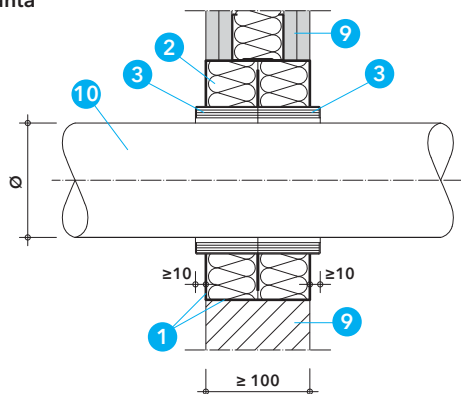
Detail O - průstup plastového potrubí ve stěnách 2) - zapuštěná varianta
