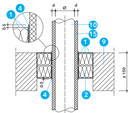
Detail T - průstup plastového izolovaného potrubí ve stropě 2)
