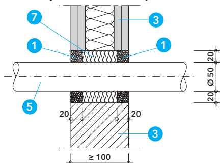
Detail I - prostup plastového potrubí podle tabulky 5 v lehké přídce nebo masivní stěně
