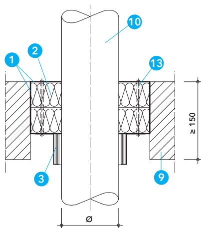
Detail N - průstup plastového potrubí ve stropěch 2) - přisazená varianta
