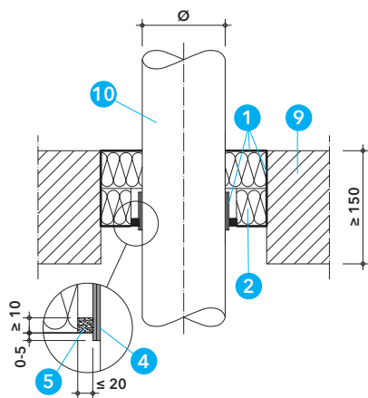
Detail S - průstup plastového potrubí ve stropě 2)
