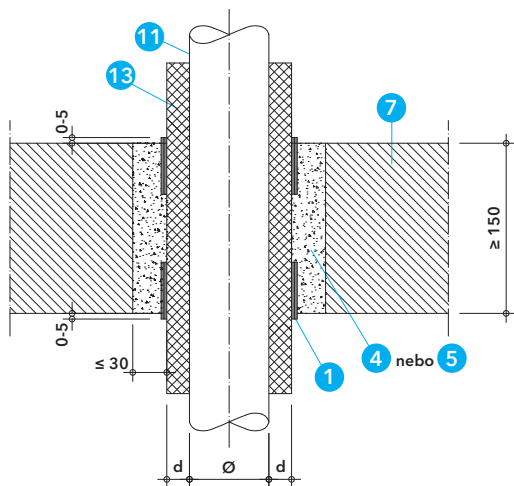
Detail J - prostup kompozitního potrubí s izolací a pásem PROMASTOP®-W ve strozech
