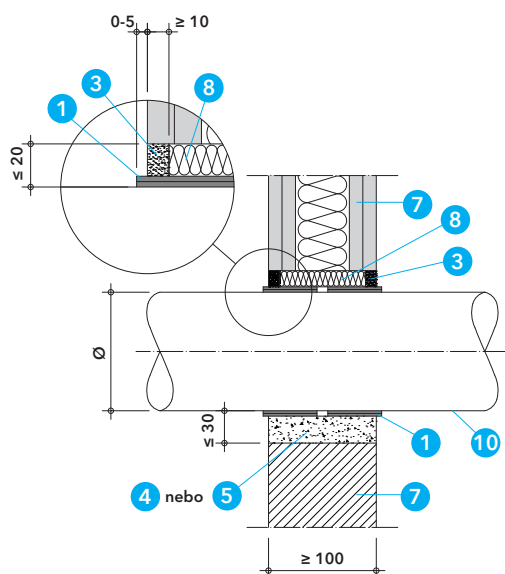
Detail B - průstup plastového potrubí s pásem PROMASTOP®-W v lehké příčce nebo masivní stěně
