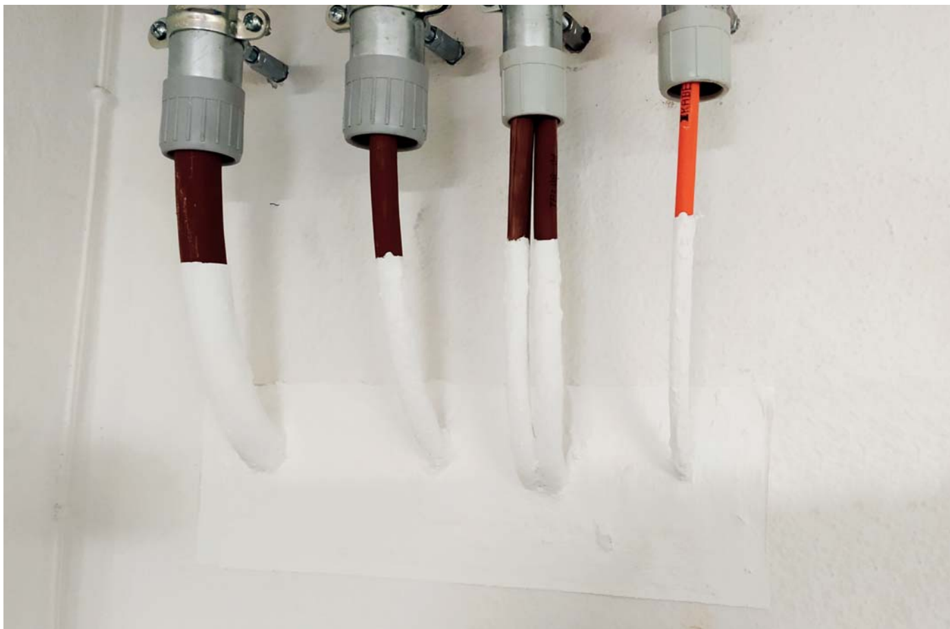
Kabelová měkká desková přepážka se stěrkou PROMASTOP®-I
