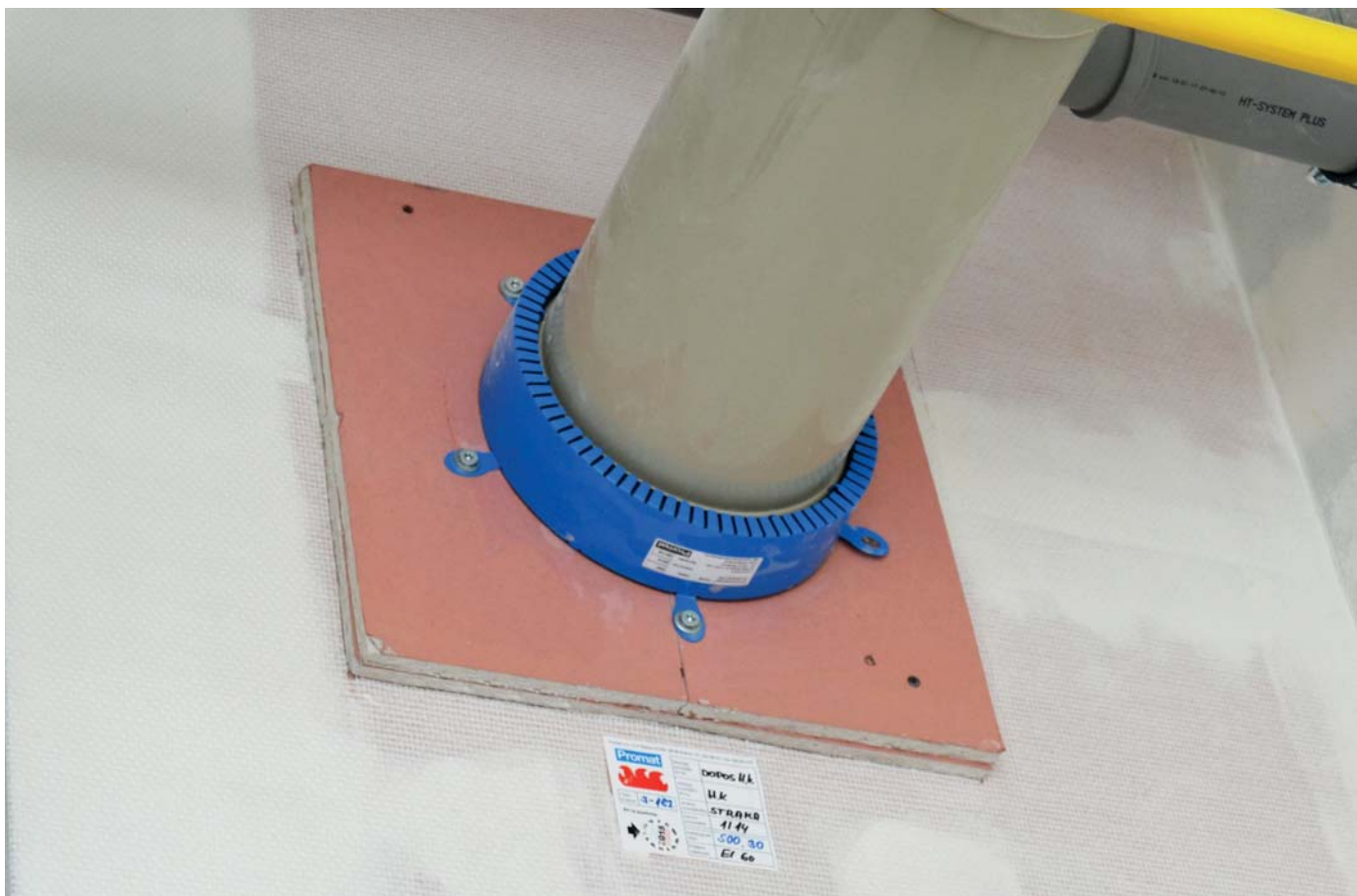
Požární ochranná manžeta PROMASTOP®-FC pro požární utěsnění plastového potrubí
