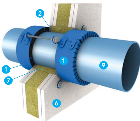
Detail B - prostup plastového potrubí s přisazenými manžetami PROMASTOP®-FC v lehké příčce
