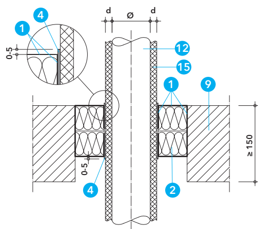
Detail V - prostup kompozitního potrubí ve stropích 2)
