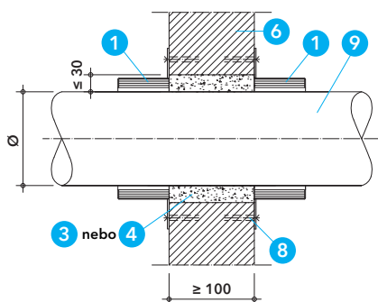
Detail E - průstup plastového potrubí v masivní stěně s manžetami PROMASTOP®-FC a maltou PROMASTOP®-M, popř. tmelem PROMATMEL®
