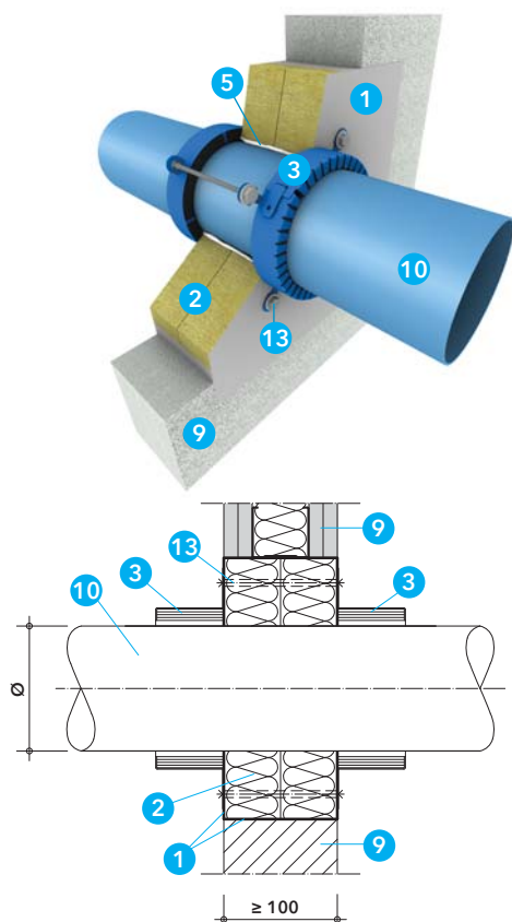
Detail M - průstup plastového potrubí ve stěnách 2) - přisazená varianta
