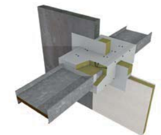
Detail Z - prostup s izolací z desek z minerální vlny
