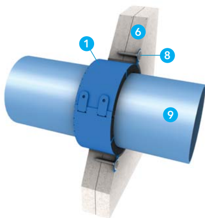
Detail C - prostup plastového potrubí s manžetou PROMASTOP®-FC v šachtové příčce
