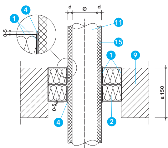
Detail X - prostup kompozitního potrubí ve stropě 2)
