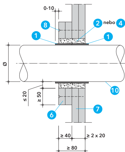
Detail A - průstup plastového potrubí s pásem PROMASTOP®-W v šachtové příčce
