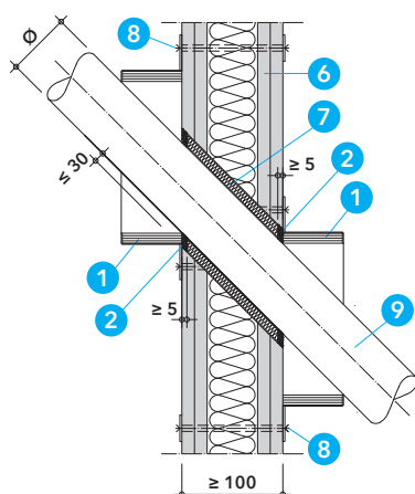
Detail X - průstup plastového potrubí v lehké přičce s manžetou PROMASTOP®-FC
