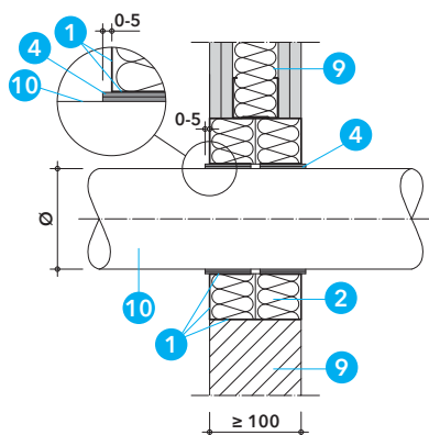
Detail R - průstup plastového potrubí ve stěnách 2)
