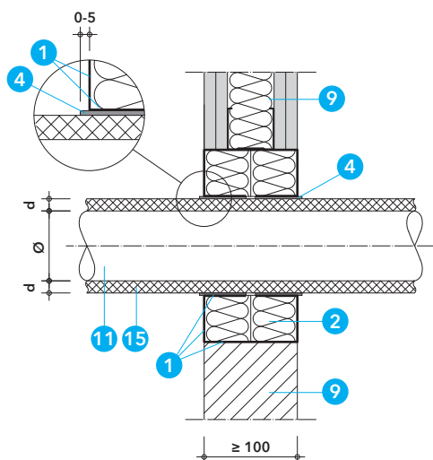
Detail W - prostup kompozitního potrubí ve stěnách 2)
