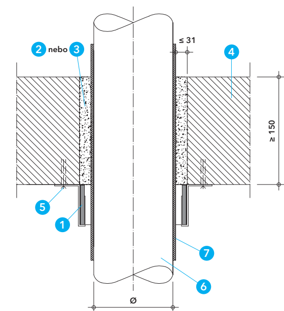
Detail B - prostup plastového potrubí s manžetou PROMASTOP®-FC MD v masivním stropě
