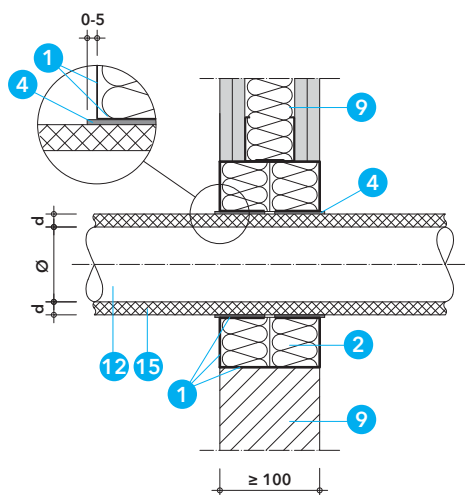
Detail U - prostup kompozitního potrubí ve stěnách 2)
