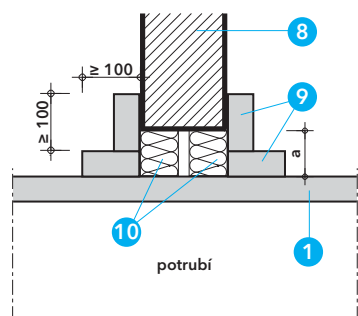
Detail B – prostup potrubí stěnou
