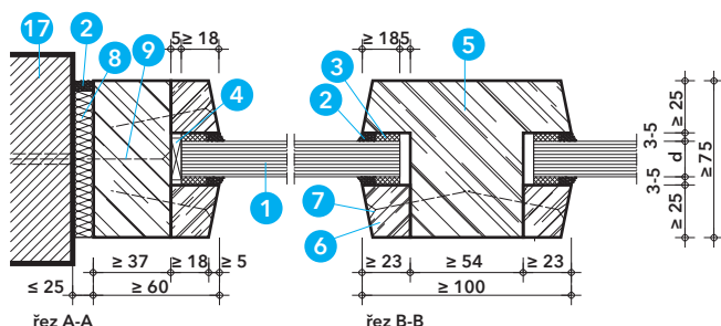
Detail B - řez rámem a připevnění k masivní konstrukci (≤ EI 45)
