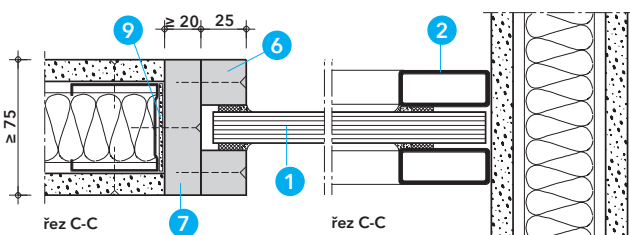
Detail E - připojení k lehkým příčkám
