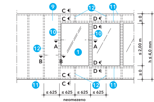
Detail A - pohled
