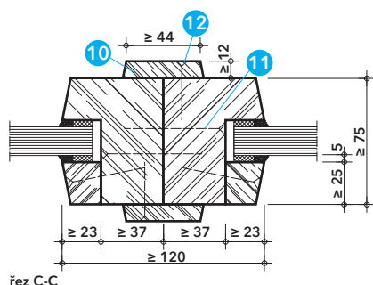
Detail D - spojení dvou ráků (≤ EI 45)
