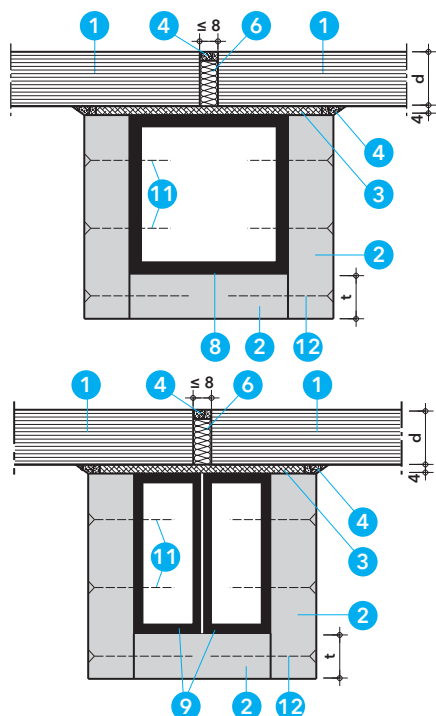
Detail B - středový profil (alternativy)
