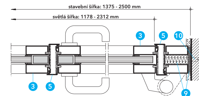
Detail D - vodorovný řez A-A
