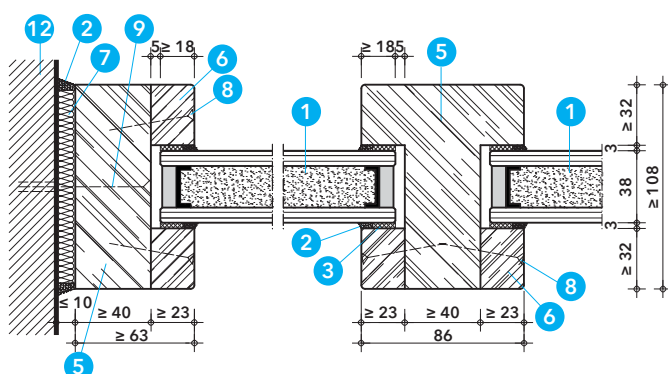
řez A-A (EI 45)
