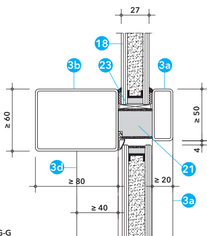
řez G-G
