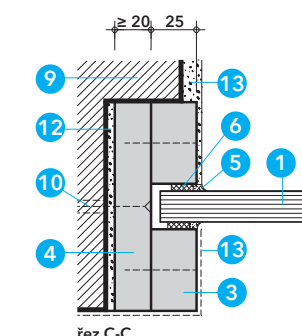
Detail E - připojení ke stěně
