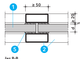
Detail D - vodorovný řez
