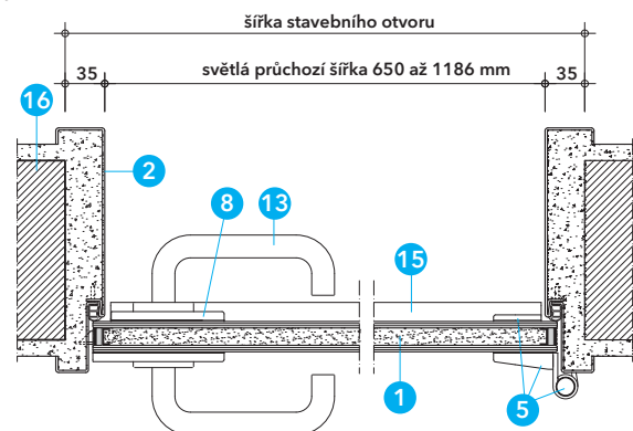
Detail B - vodorovný řez A-A - jednokřídlé dveře
