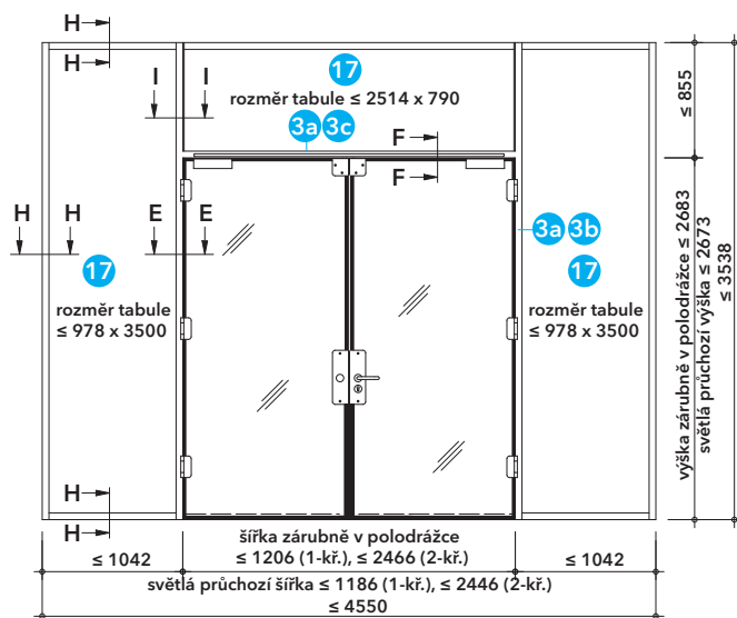
Detail F - jednokřídlé a dvoukřídlé dveře s bočními světílkami a nadsvětlíkem - varianta A
