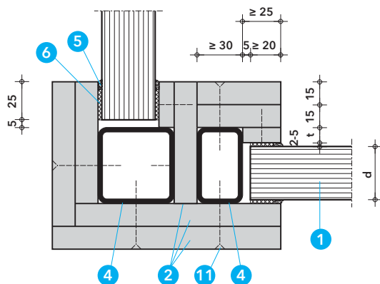
Detail E - rohové spojení 90°
