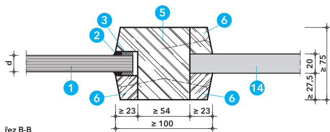
Detail H - plná výplň PROMATECT®-H (≤ EI 30/EW 45)
