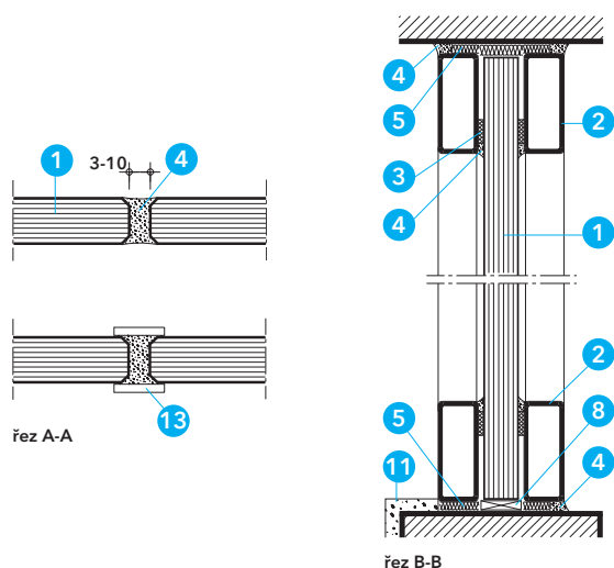
Detail B - spára mezi skly
