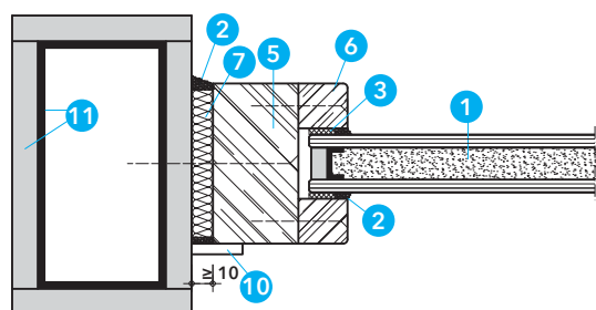
řez A-A
