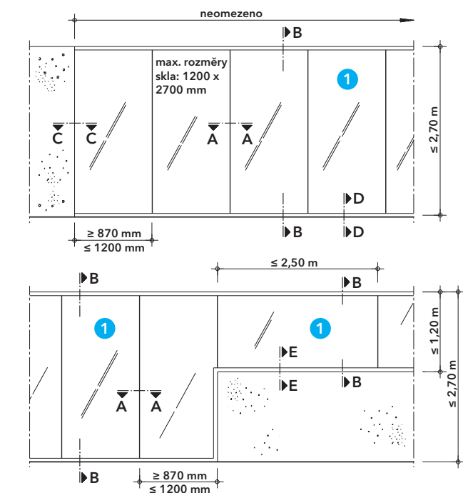
Detail A - rozměry
