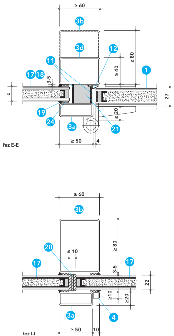
Detail G - jednokřídlé a dvoukřídlé dveře s bočními světlíky a nadsvětříkem - varianta A
