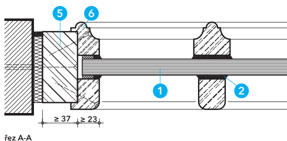
Detail G - varianty dřevěných lišt (≤ EI 45)
