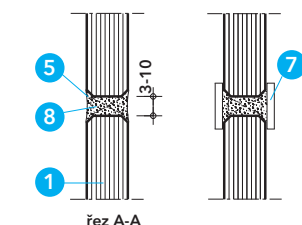
Detail C - spáry mezi skly
