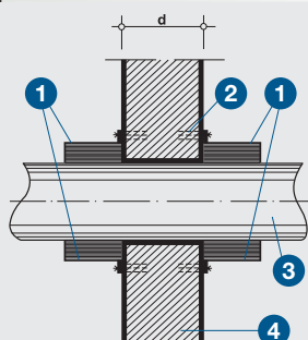
Detail A – průchod stěnou
