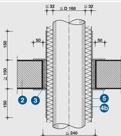
Detail D – prostup potrubí s tepelnou (zvuk.) izolací stropem EI 90 U/C
