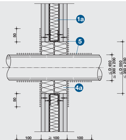
Detail C – prostup potrubí bez izolace stěnou EI 120 U/C, EI 120 C/U
