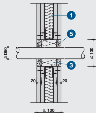
Detail A – vstup plastového potrubí stěnou EI 90 U/C, EI 90 C/U
