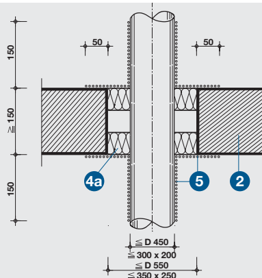
Detail F – prostup potrubí bez izolace stropem EI 120 U/C
