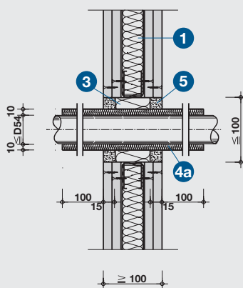
Detail B – vstup kov. potrubí do D 50 mm stěnou EI 120 U/C, EI 120 C/U
