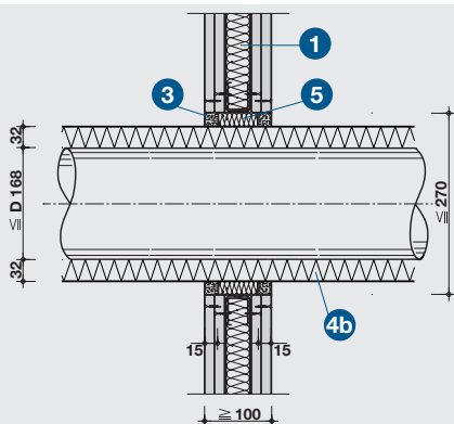
Detail D – vstup kov. potrubí s tepelnou (zvuk.) izolací stěnou EI 90 U/C
