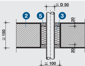
Detail E – vstup plastového potrubí stropem
