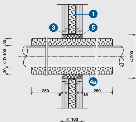
Detail C – vstup kov. potrubí do D 106 mm stěnou EI 120 U/C, EI 120 C/U
