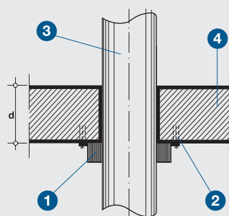
Detail B – průchod stropem
