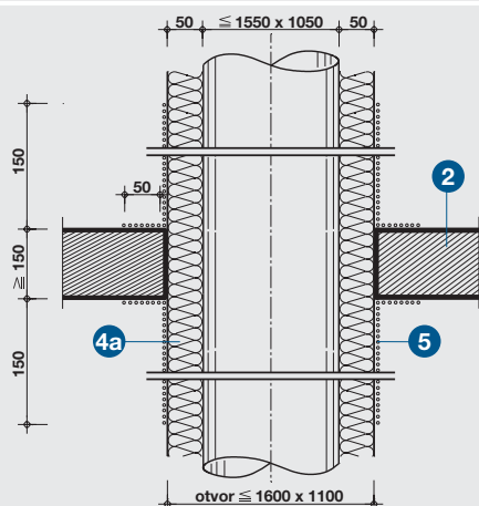
Detail E – prostup potrubí s izolací stropem EI 90 U/C
