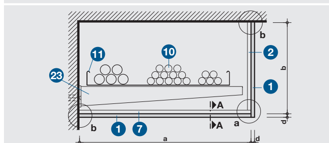
Detail A.2 – příčný řez
