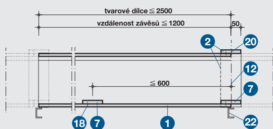
Detail B – podélný řez
