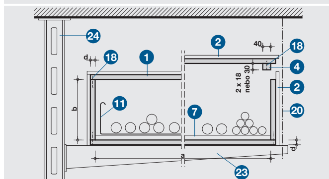
Detail A.1 – příčný řez
