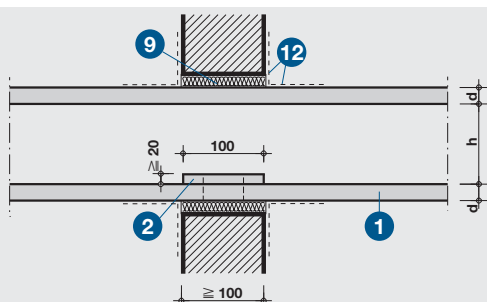
Detail D – průchod kabelového kanálu se stěrkou PROMASTOP®-P
