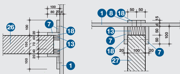
Detail E.3 – prostup instalačního kanálu masivní stěnou
