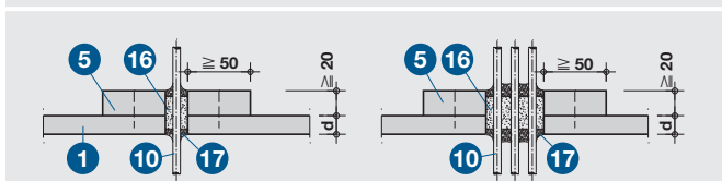
Detail I – vyvedení kabelů
