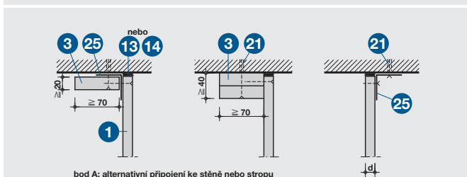
Detail G – detaily připojení
