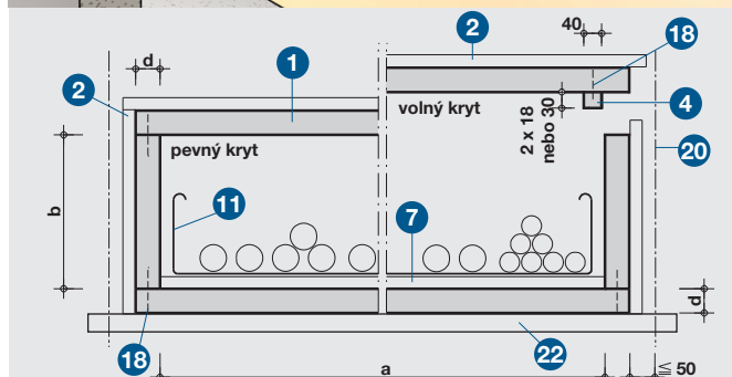
Detail A – příčný řez kabelovým kanálem
